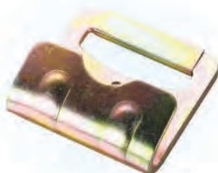
HYFH-077 A=70mm B=98mm C=5mm PULL≤6800KG
